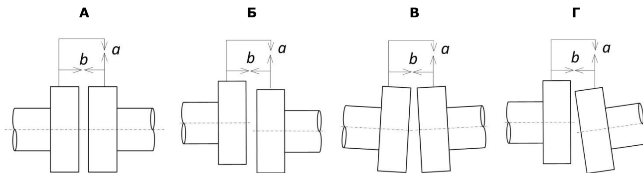
Рисунок 8. Возможные взаимные положения валов
