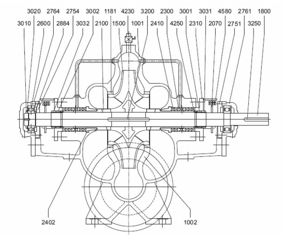
Рисунок 22. Поперечный разрез стандартного одноступенчатого насоса SCP с сальниковым уплотнением
