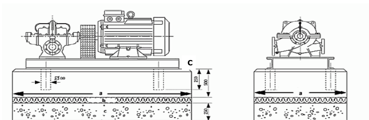
Рисунок 3. Пример фундамента
