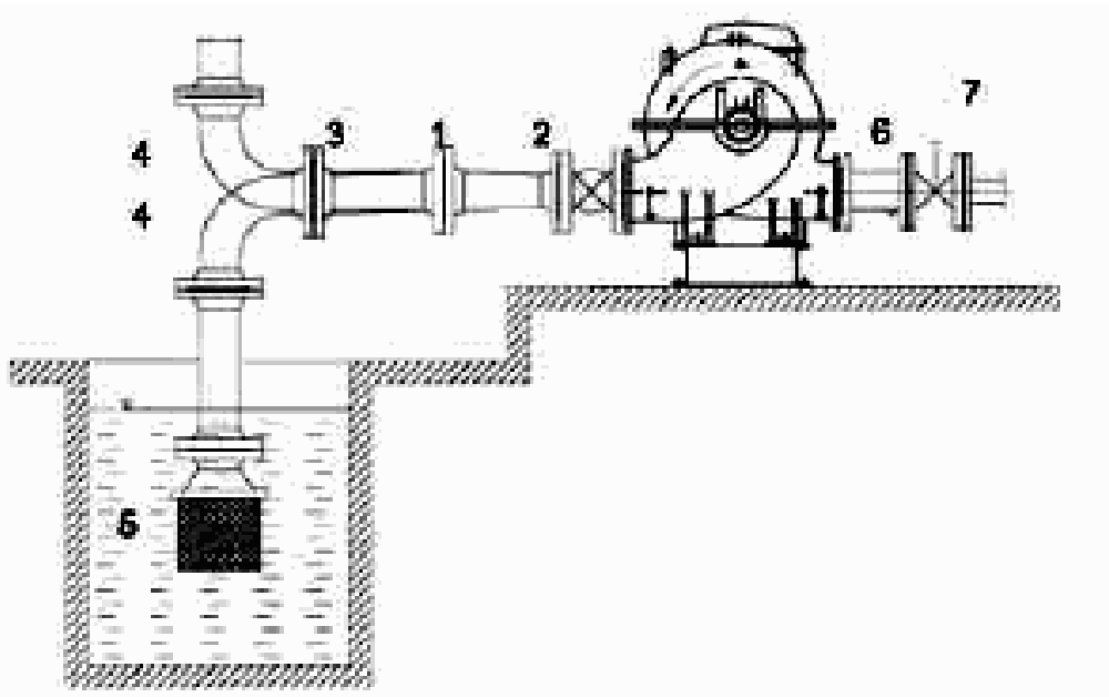
Рисунок 18. Расположение насоса
