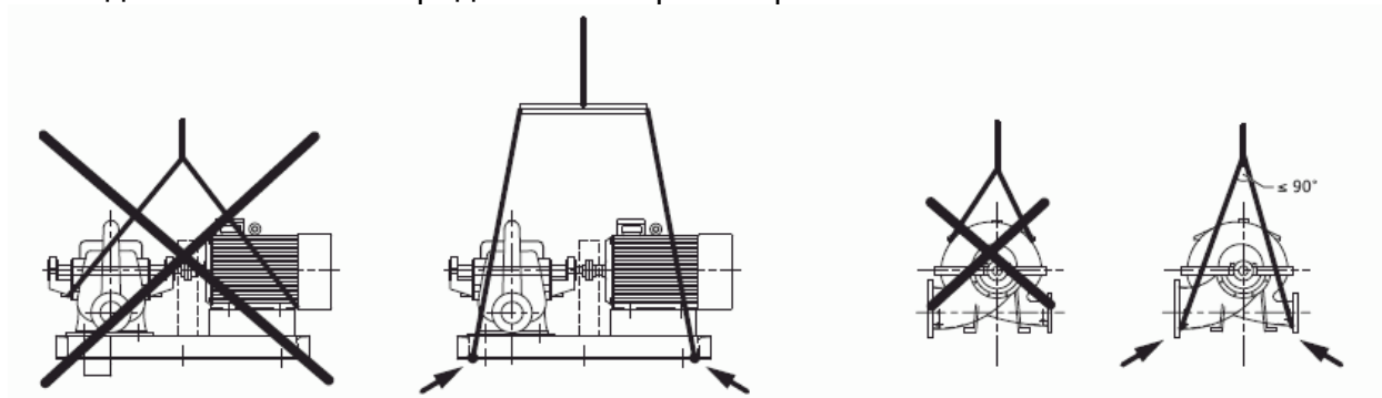
Рисунок 1а. Обращение с горизонтальным насосом SCP при погрузке и транспортировке
