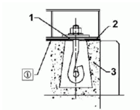
Рисунок 5. Фундаментный болт
