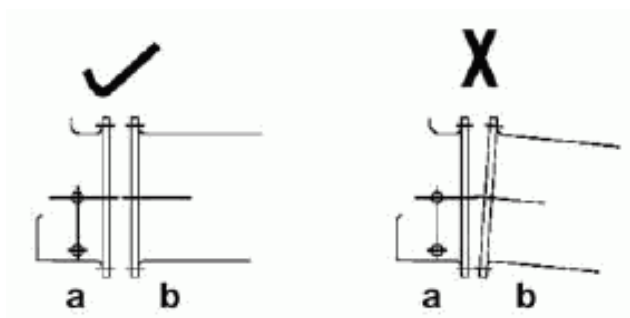
Рисунок 10. Крепление трубопровода к фланцам насоса а: фланец насоса; b: трубопровод
