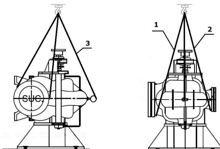
Рисунок 1а. Обращение с горизонтальным насосом SCP при погрузке и транспортировке
