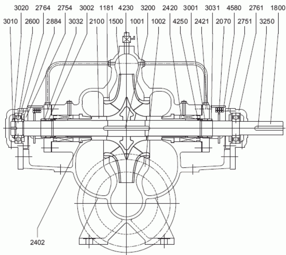
Рисунок 21. Поперечный разрез стандартного одноступенчатого насоса SCP с торцевым уплотнением.
