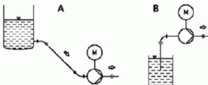
Рисунок 12. Расположение насоса
