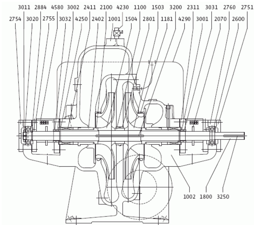
Рисунок 23. Поперечный разрез стандартного двухступенчатого насоса SCP с торцевым уплотнением
