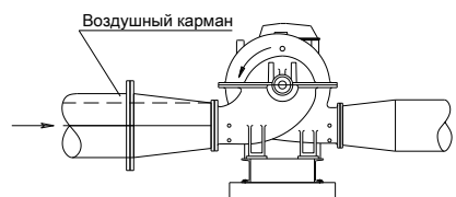
Рисунок 13. Конструкция всасывающего трубопровода
