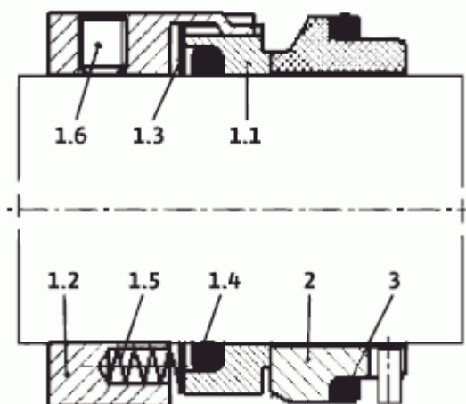
Рисунок 2. Торцевое уплотнение
