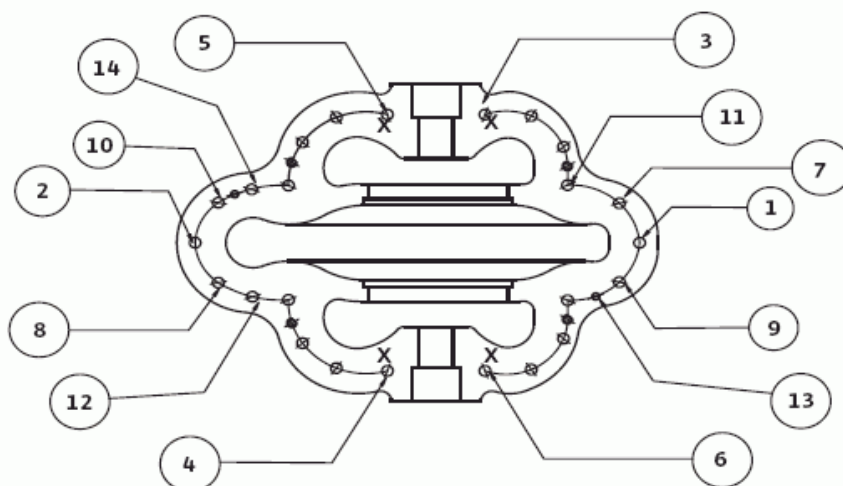
Рисунок 20. Повторная сборка: порядок затяжки болтов
