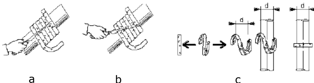
Рисунок 19. Набивка сальника
