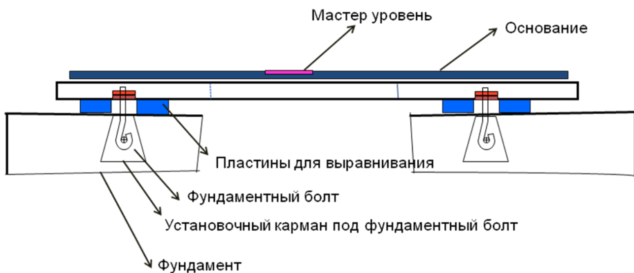
Рисунок 4. Выравнивание фундаментной плиты
