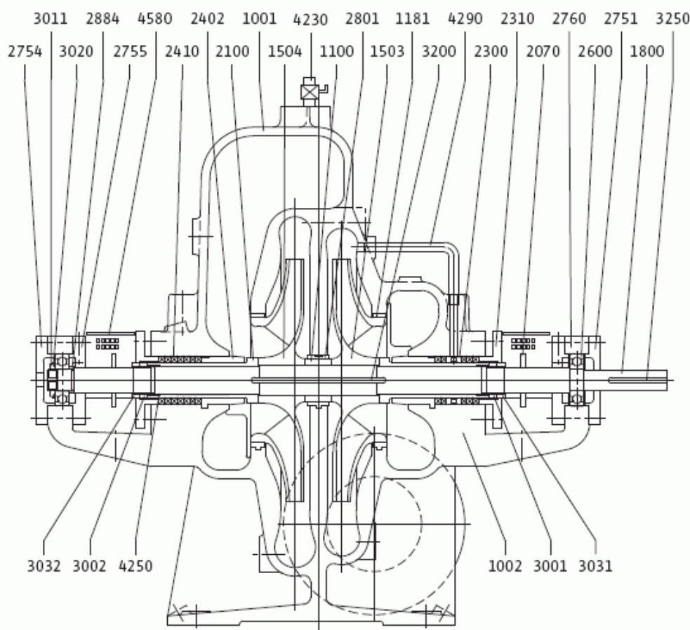
Рисунок 24. Поперечный разрез стандартного двухступенчатого насоса SCP с сальниковым уплотнением
