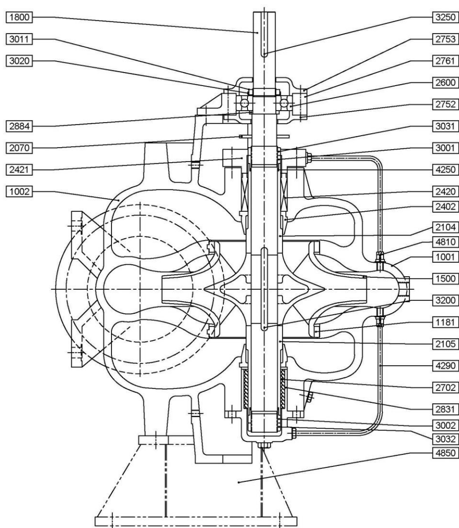
Рисунок 25. Поперечный разрез стандартного одноступенчатого насоса SCPV с торцевым уплотнением
