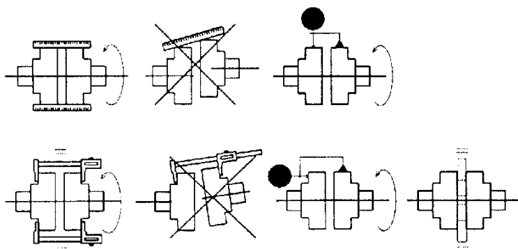
Рисунок 7. Центрирование валов насоса и мотора
